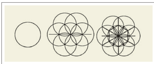
تصویر ۱۸: روش سنتی رسم شش ضلعی (مأخذ: بروگ، ۱۲۸۷، ۱۹)
