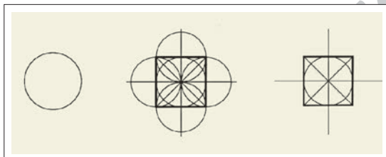
■ تصویر ۱۴: روش سنتی رسم مربع از دایره، (مأخذ: بروگ، ۱۲۸۷، ۱۵)
