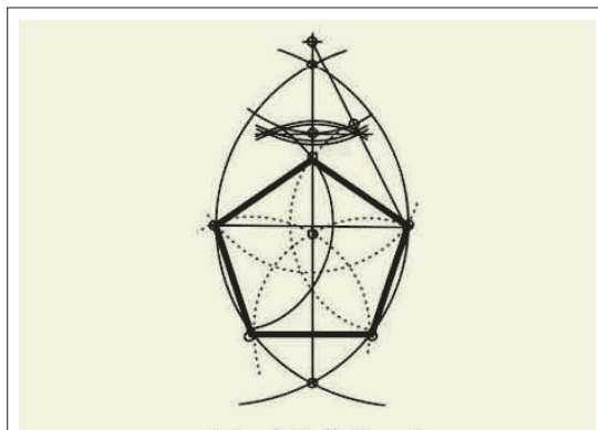
تصویر ۲۰: روش رسم پنج ضلعی منتظم با استفاده از دو کمان (مأخذ: Critchlow, 1999, 77)
